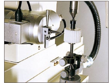
☀ 成形プラスチックギヤの測定 Measurement of plastic gear
