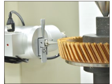
☀ ピニオンカッタの測定 Measurement of pinion (shaper) cutter
