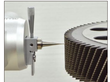
☀ シェービングカッタの測定 Measurement of shaving cutter
